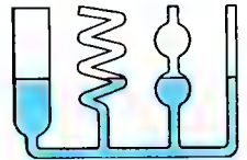
Сполучені посудини
